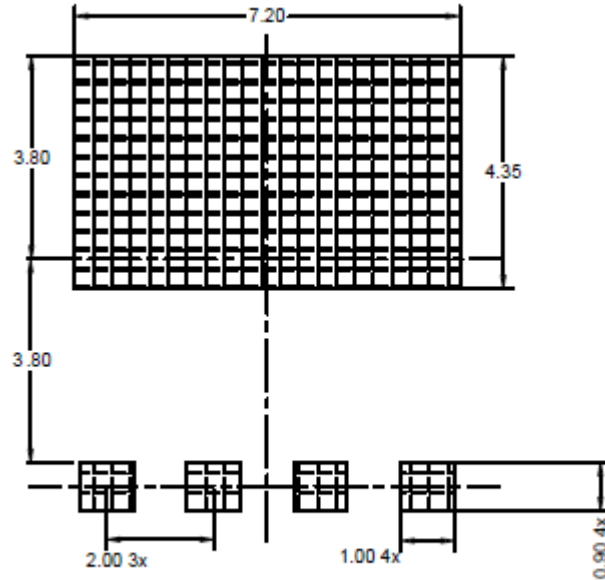
DFN 8*8-4L
