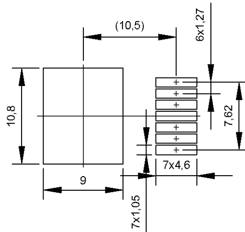
TO-263-7L
